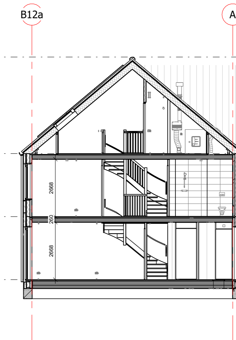
langsdoorsnede bnr 44 schaal 1:100
