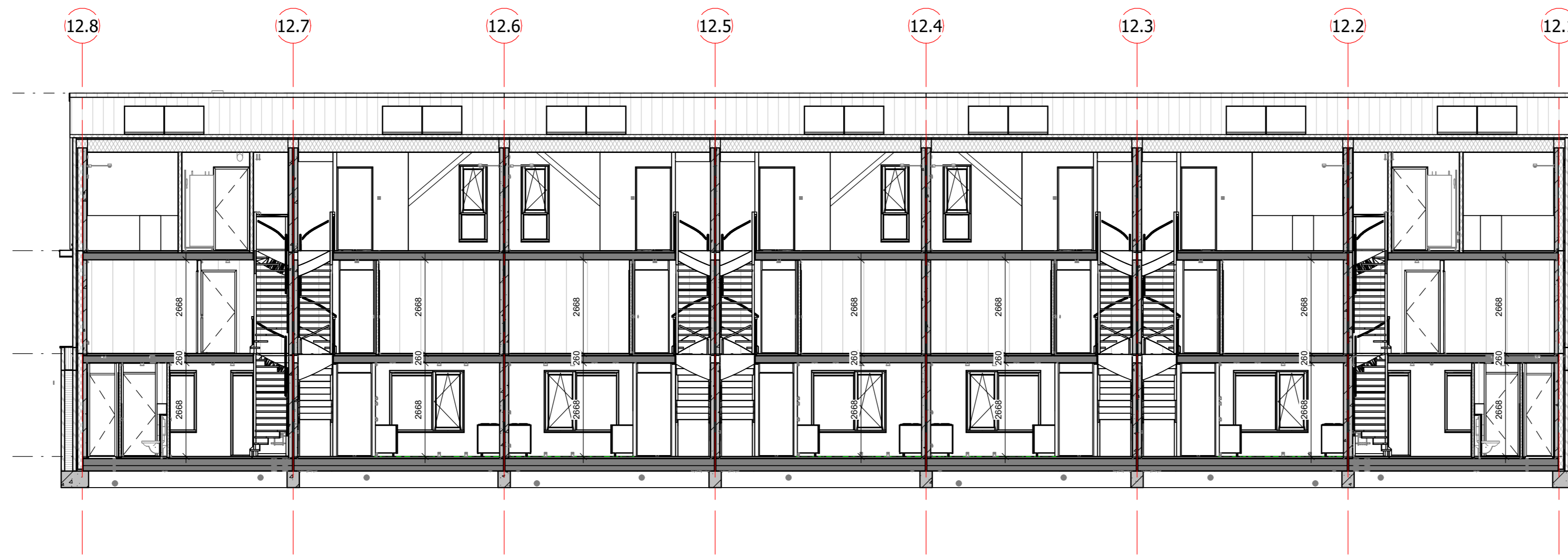
dwarsdoorsnede blok 12 schaal 1:100
