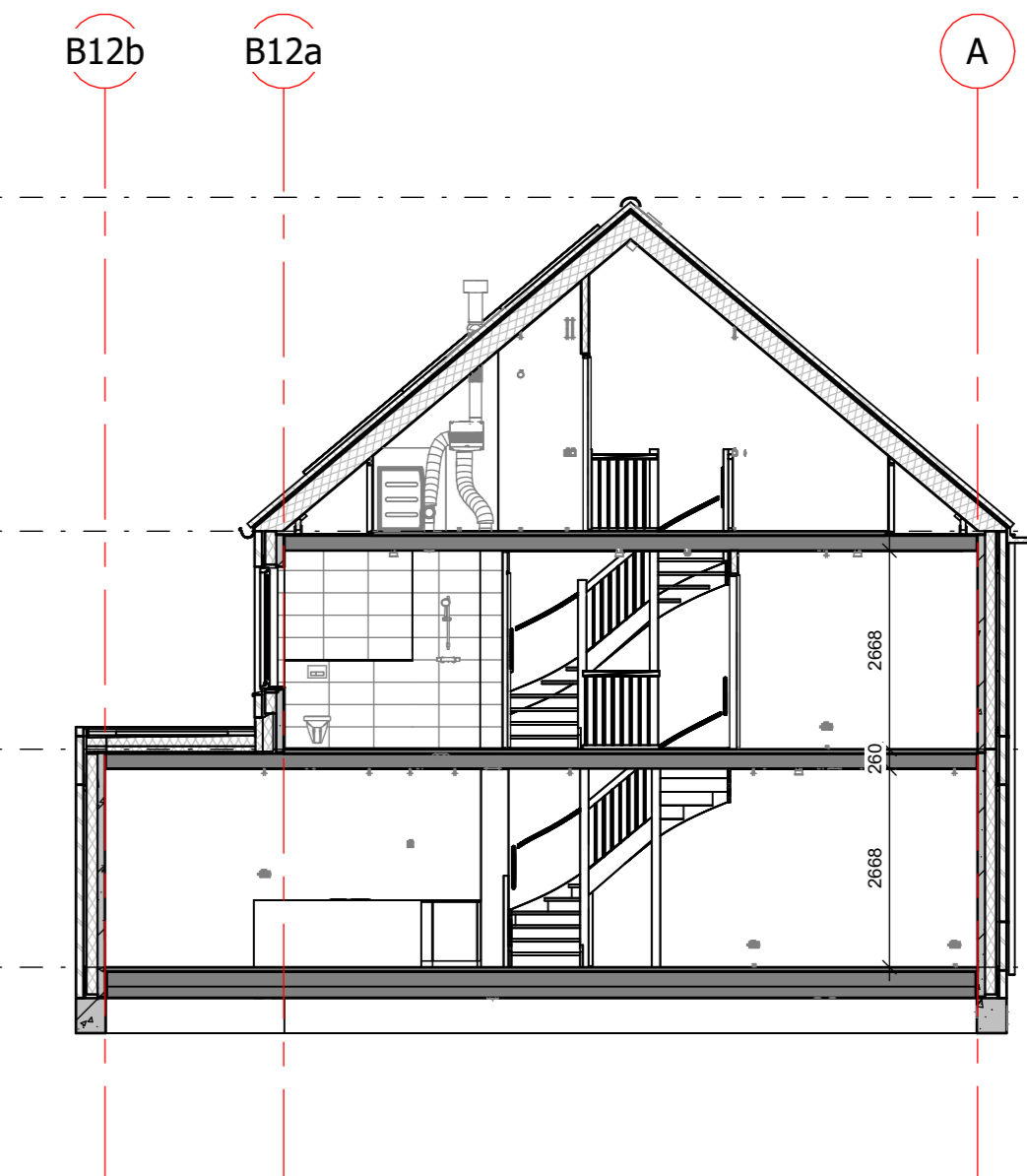
langsdoorsnede bnr 45 schaal 1:100
