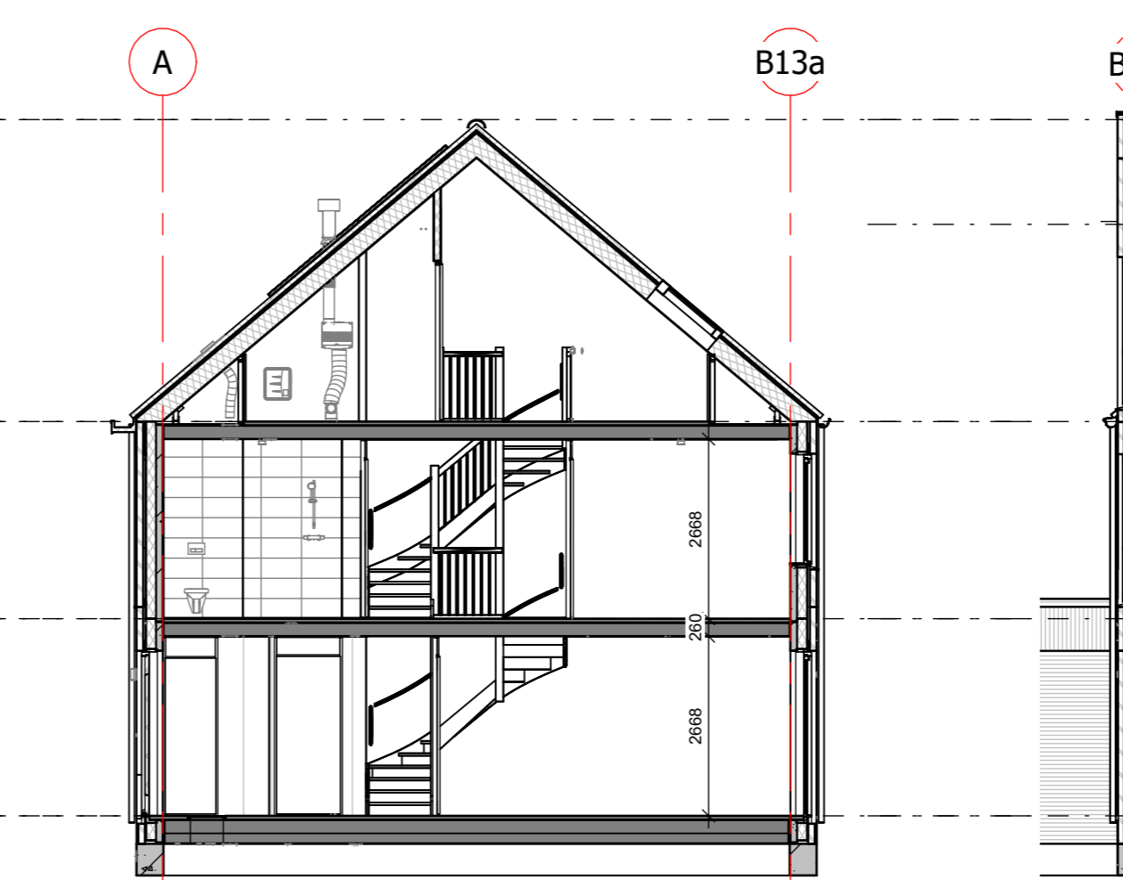
doorsnede bnr 48
