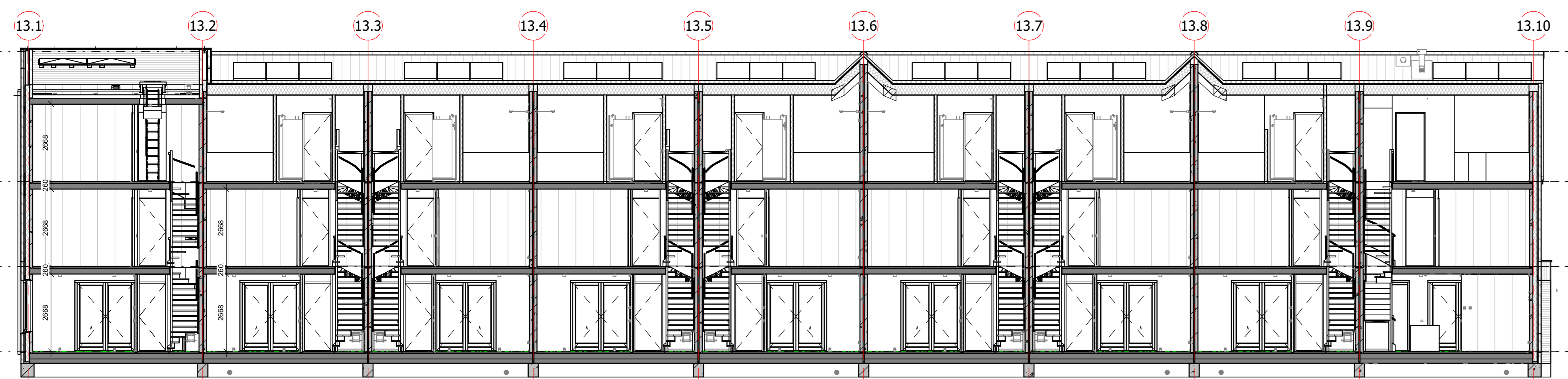
3b_doorsnede_blok_13
