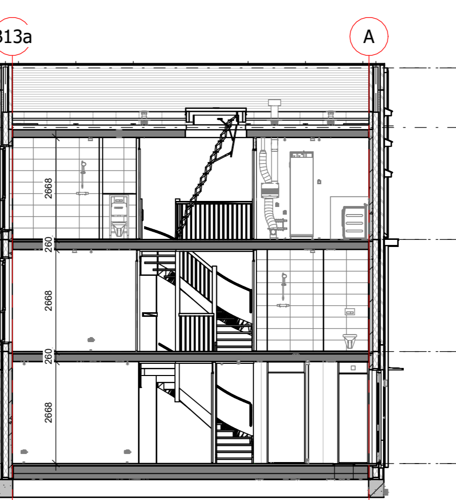
doorsnede bnr 46
