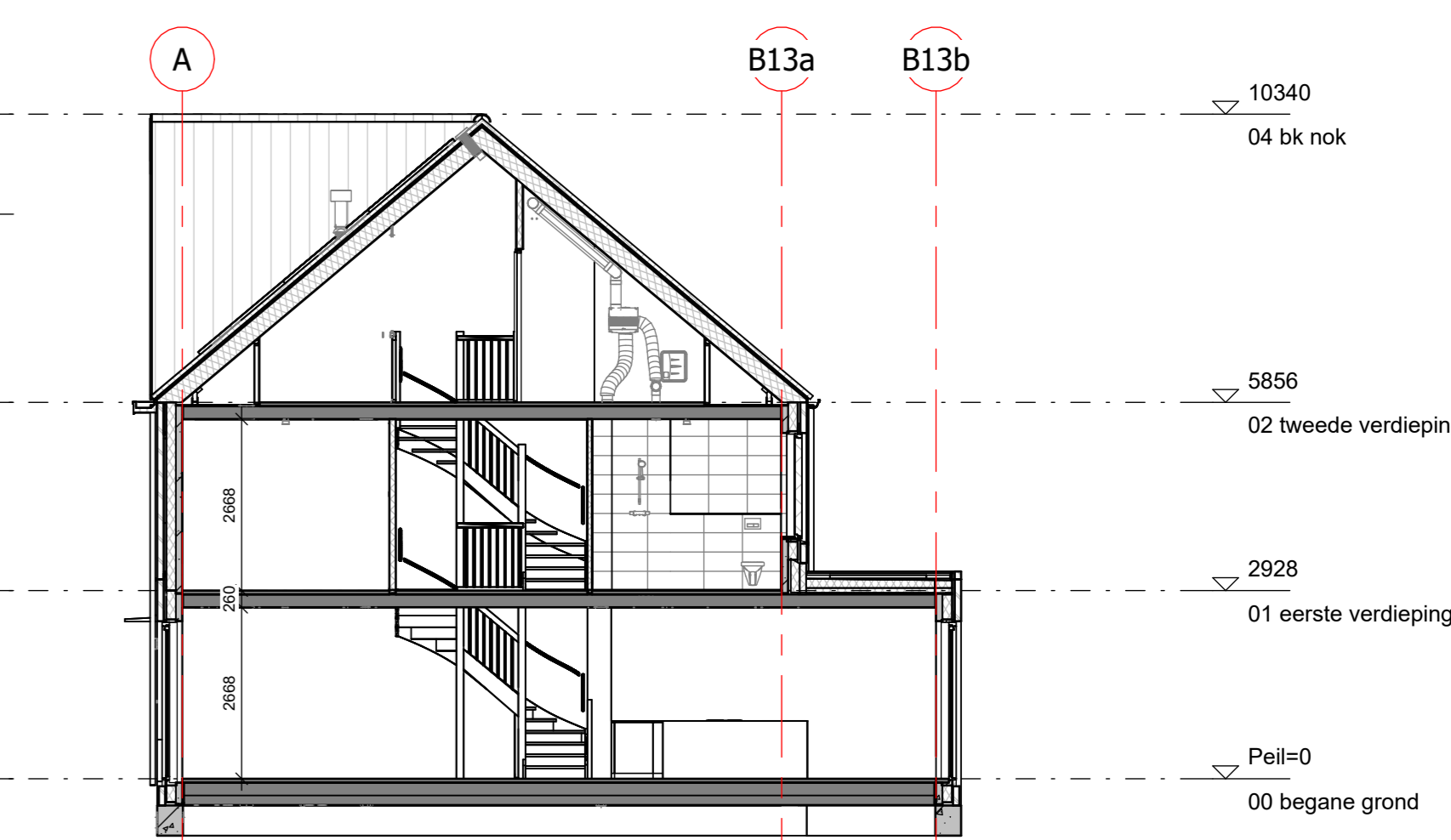
doorsnede bnr 54
